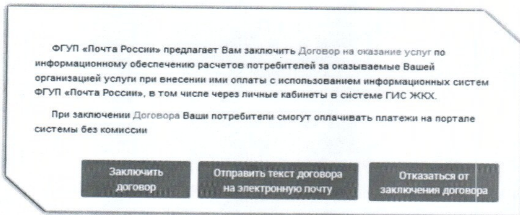
Рис. 2 Информационное окно
